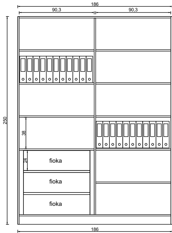
plakar sa kliznim vratima za smestaj registratora
